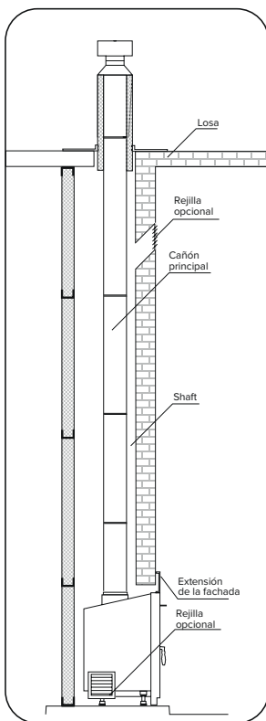
Instalación en closets existente, nicho o encuentro de muros
