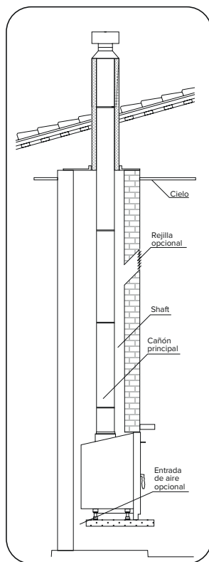
Instalación sobre loseta en altura
