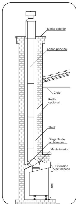
Instalación en chimeneas ya existentes
